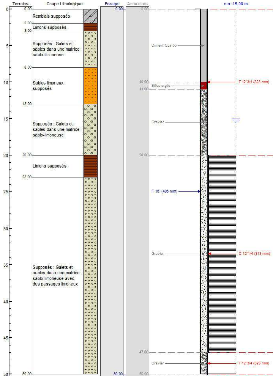
Figure 10 : Coupe géologique et technique prévisionnelle des forages de rejet
